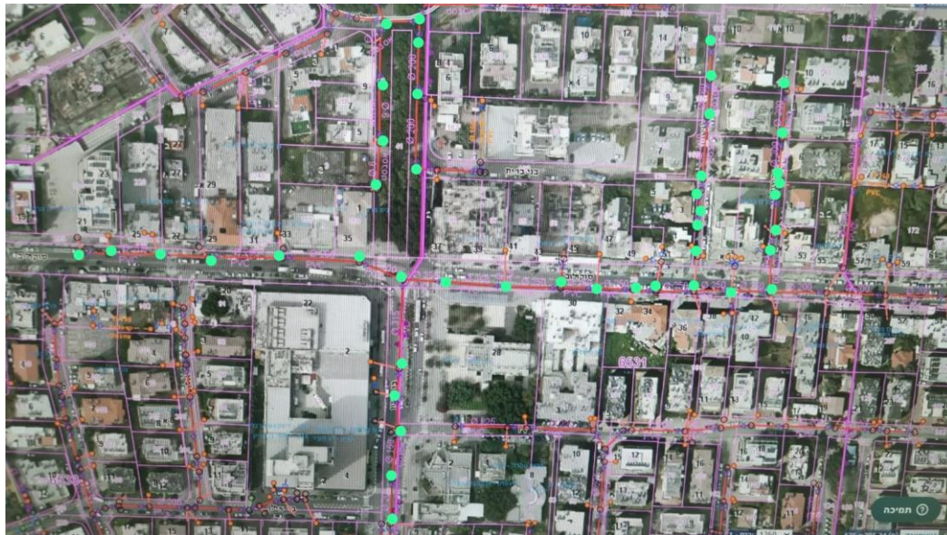
מפת שטיפת קווי ביוב ושוחות ביוב בסוקולוב
