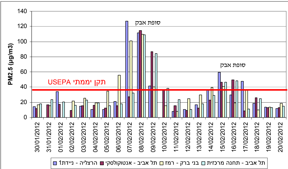
גרף 13: המהלך התקופתי של ריכוזי PM 2.5 יממתיים בניידת הניטור בהרצליה בתחנה התחבורתית בבני ברק (רמז) ובתחנות הכלליות בת"א (אנטוקולסקי ותחנה מרכזית) בין 30/01/2012 - 20/02/2012
